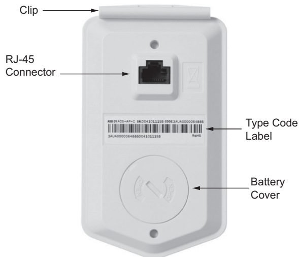
Fig. 58 — ACH580 VFD Keypad — Back
