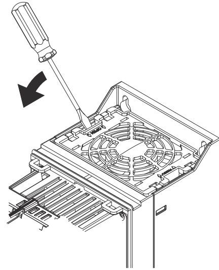
Fig. 43 — Remove Main Fan Fingerguard
